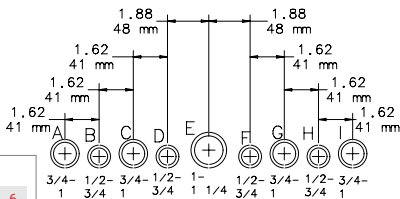
Conduit Sizes
