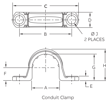
Conduit Clamp
