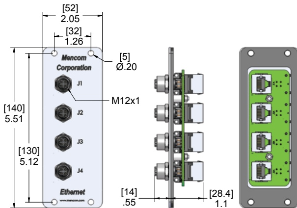
D24-4MDE45-4FR-RJ45
