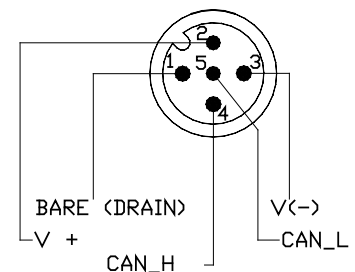
All Port Pin Wiring
