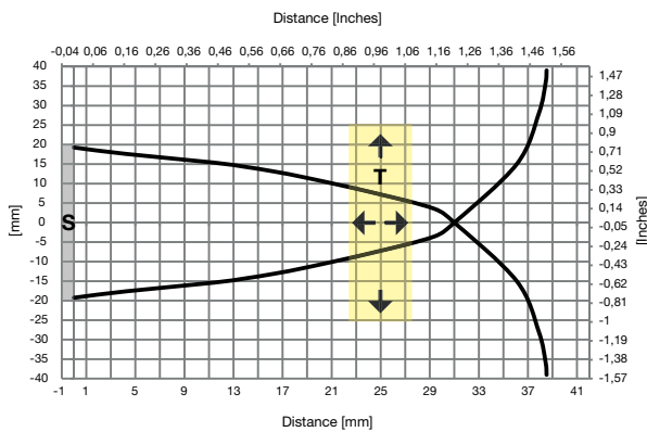
Fig. 2 Non-flush
