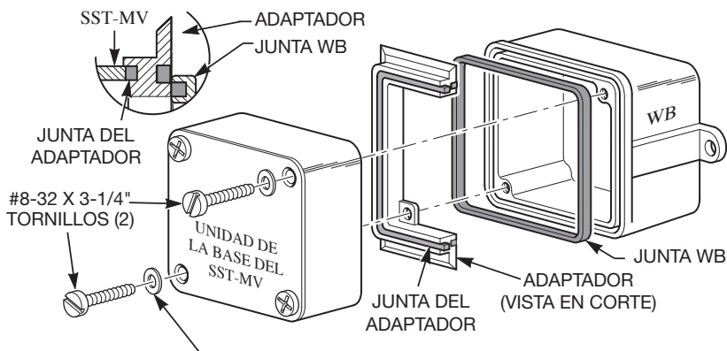
Figura 1 Montaje con la caja WB
