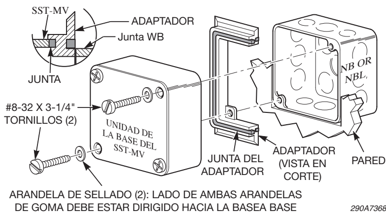
Figura 2 Montaje con una caja NB o NBL
