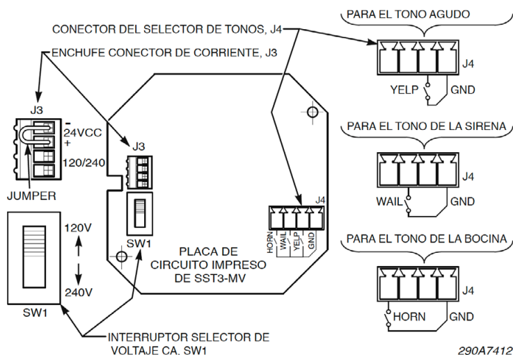
Figura 4 Ajustes de la PCB de la sirena
