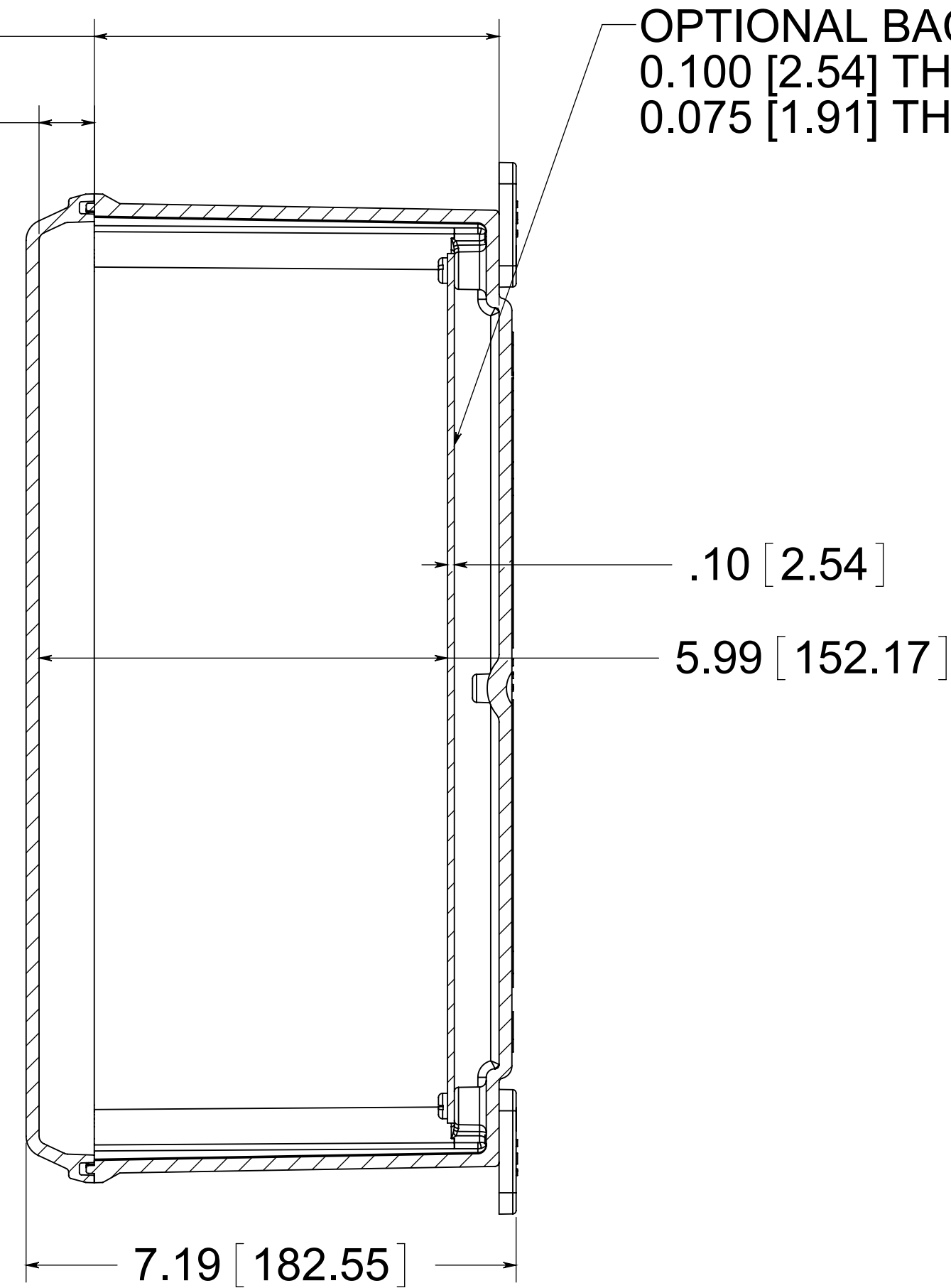
SECTION A-A
