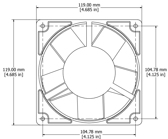
FAN TOP VIEW (2X)
