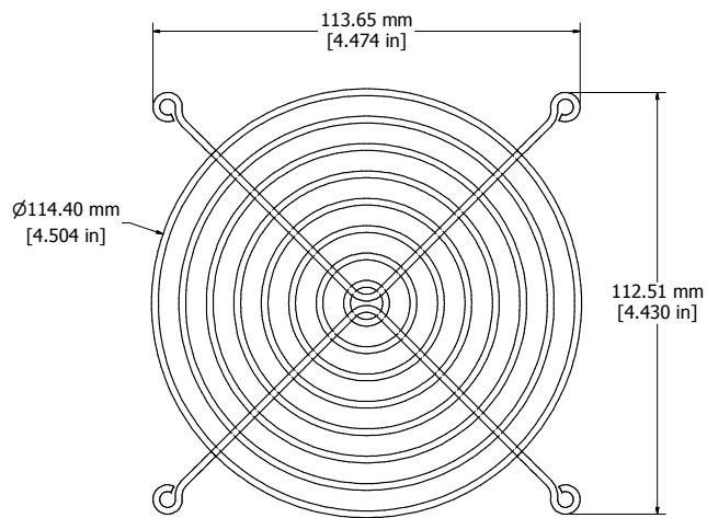
FAN GUARD TOP VIEW (4X)
