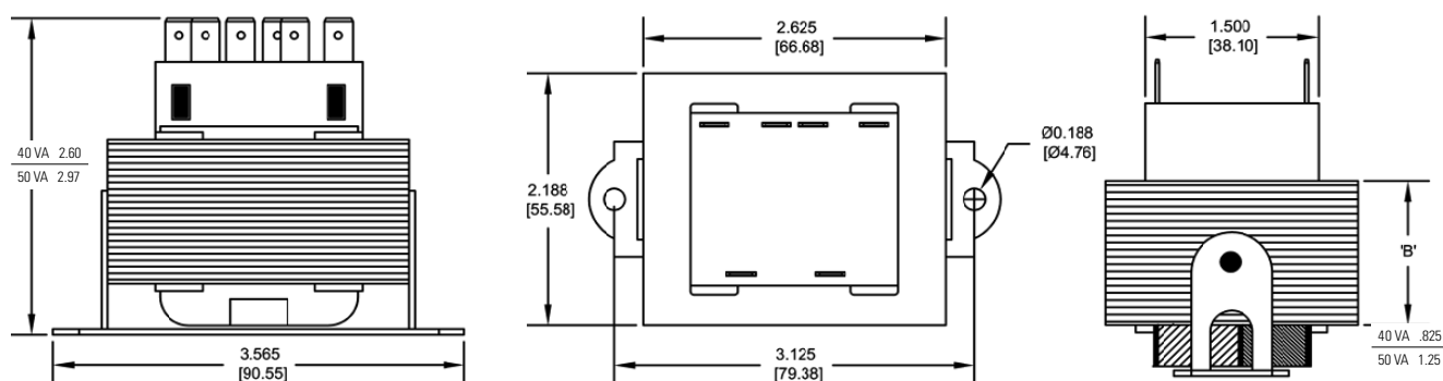
40 & 50 VA Transformer
