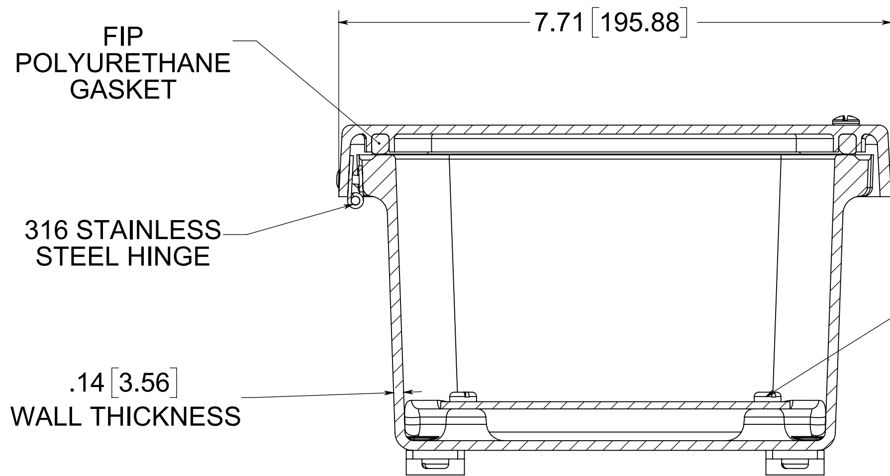
SECTION A-A
