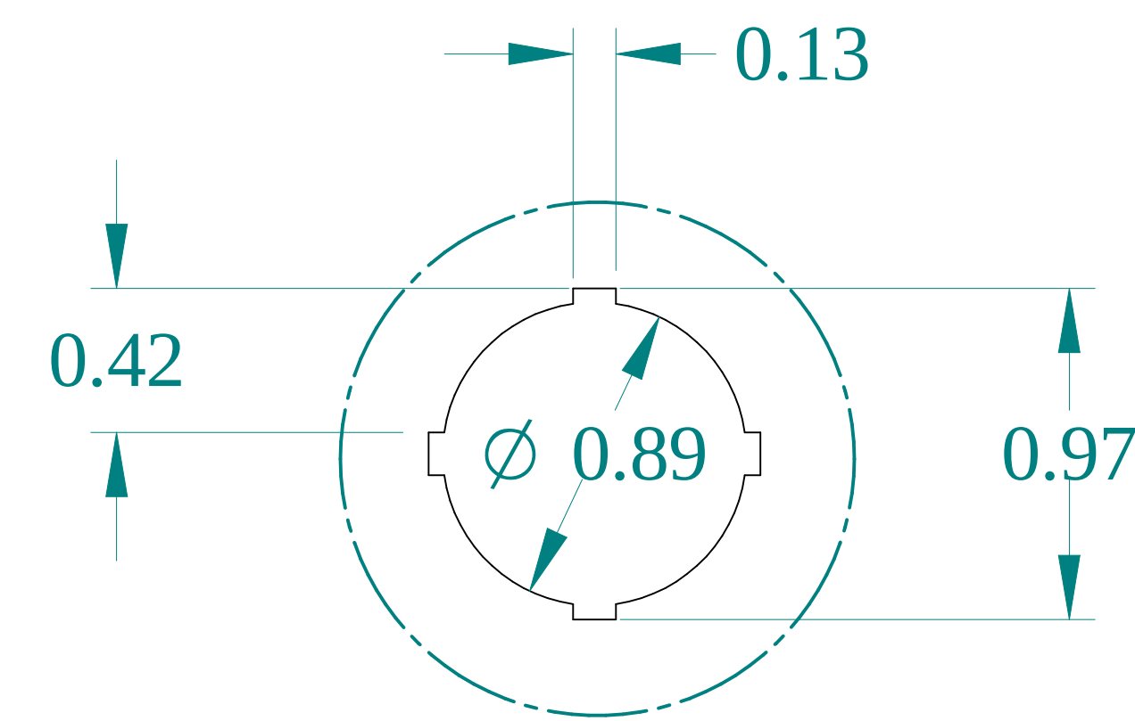
DETAIL Z TYP
