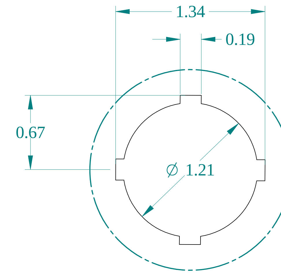
DETAIL Y
