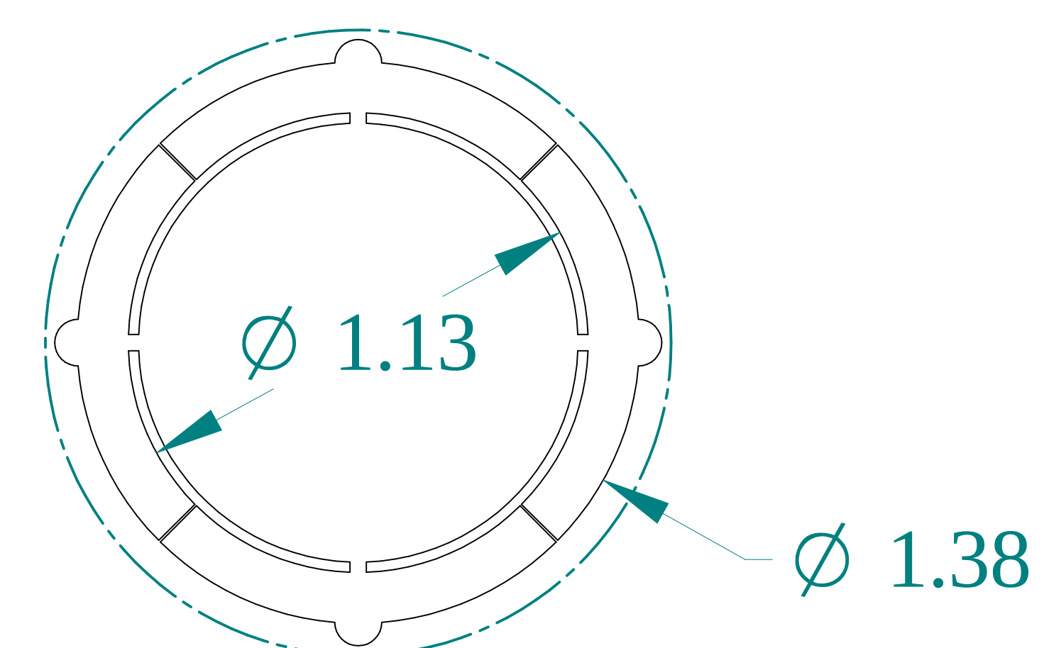
DETAIL Z TYP
