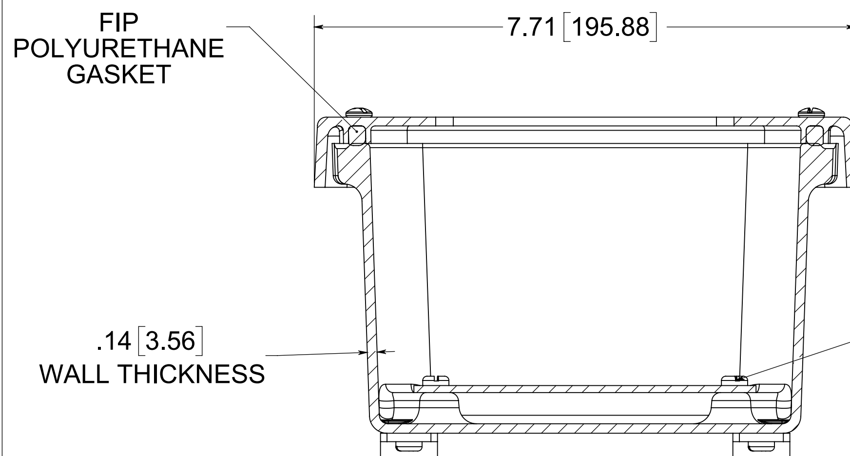
SECTION A-A
