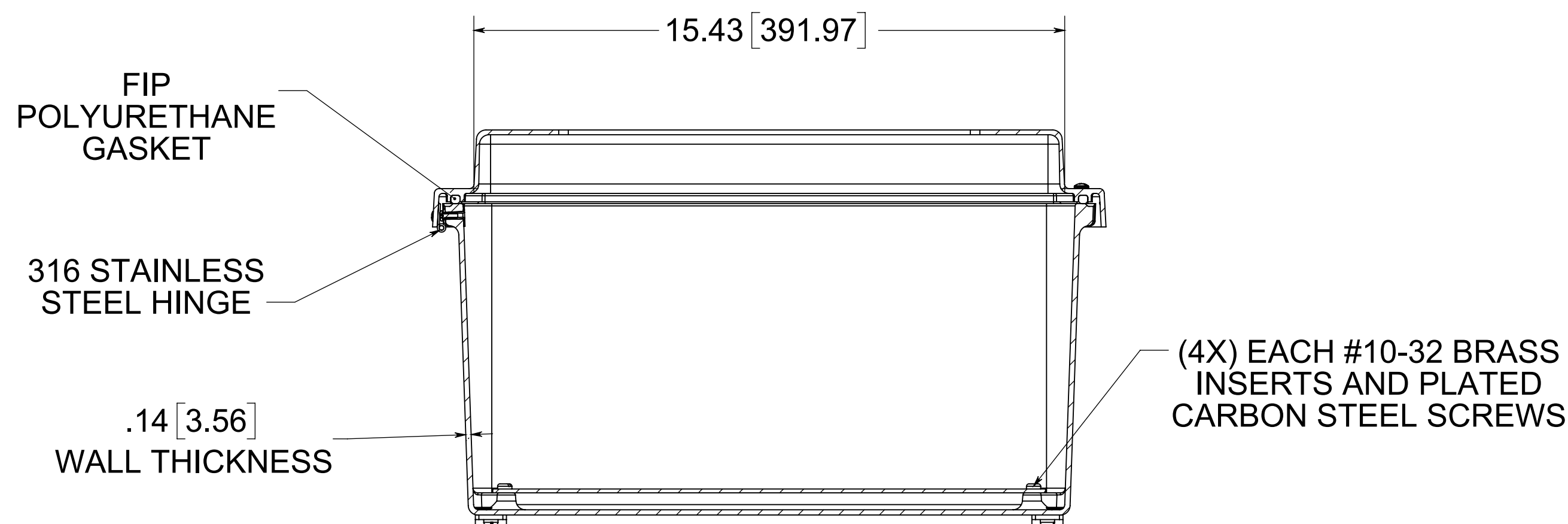
SECTION A-A
