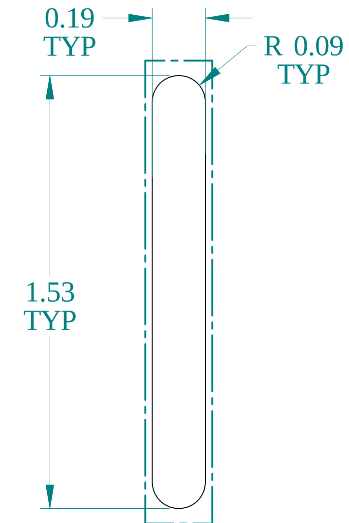
DETAIL Z TYP
