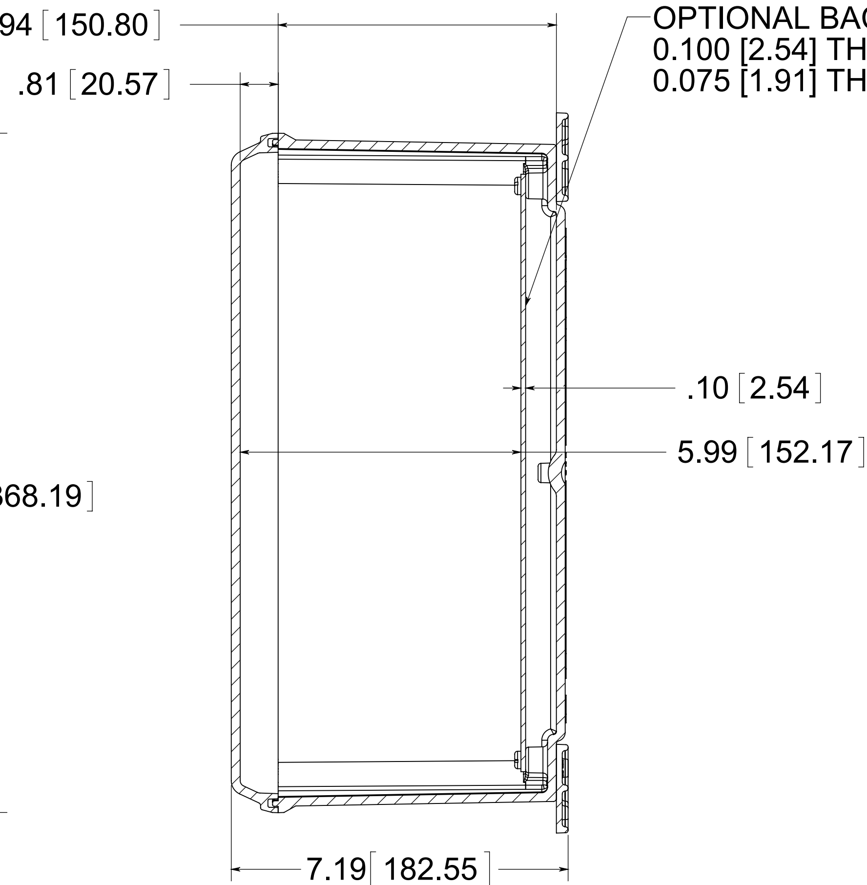
SECTION A-A
