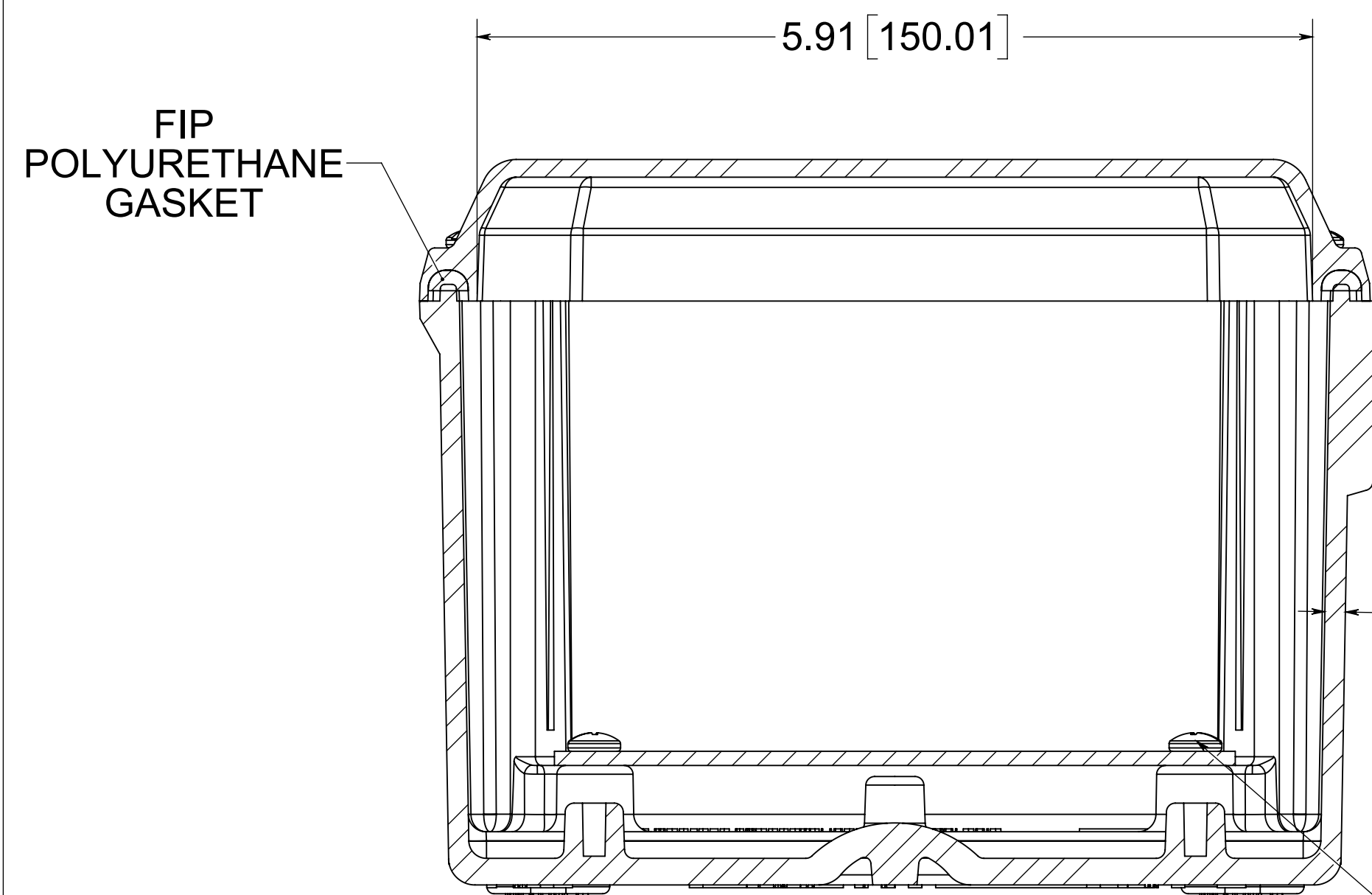
SECTION A-A
