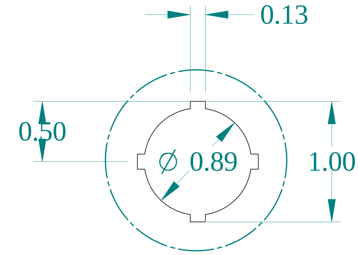
DETAIL Z TYP
