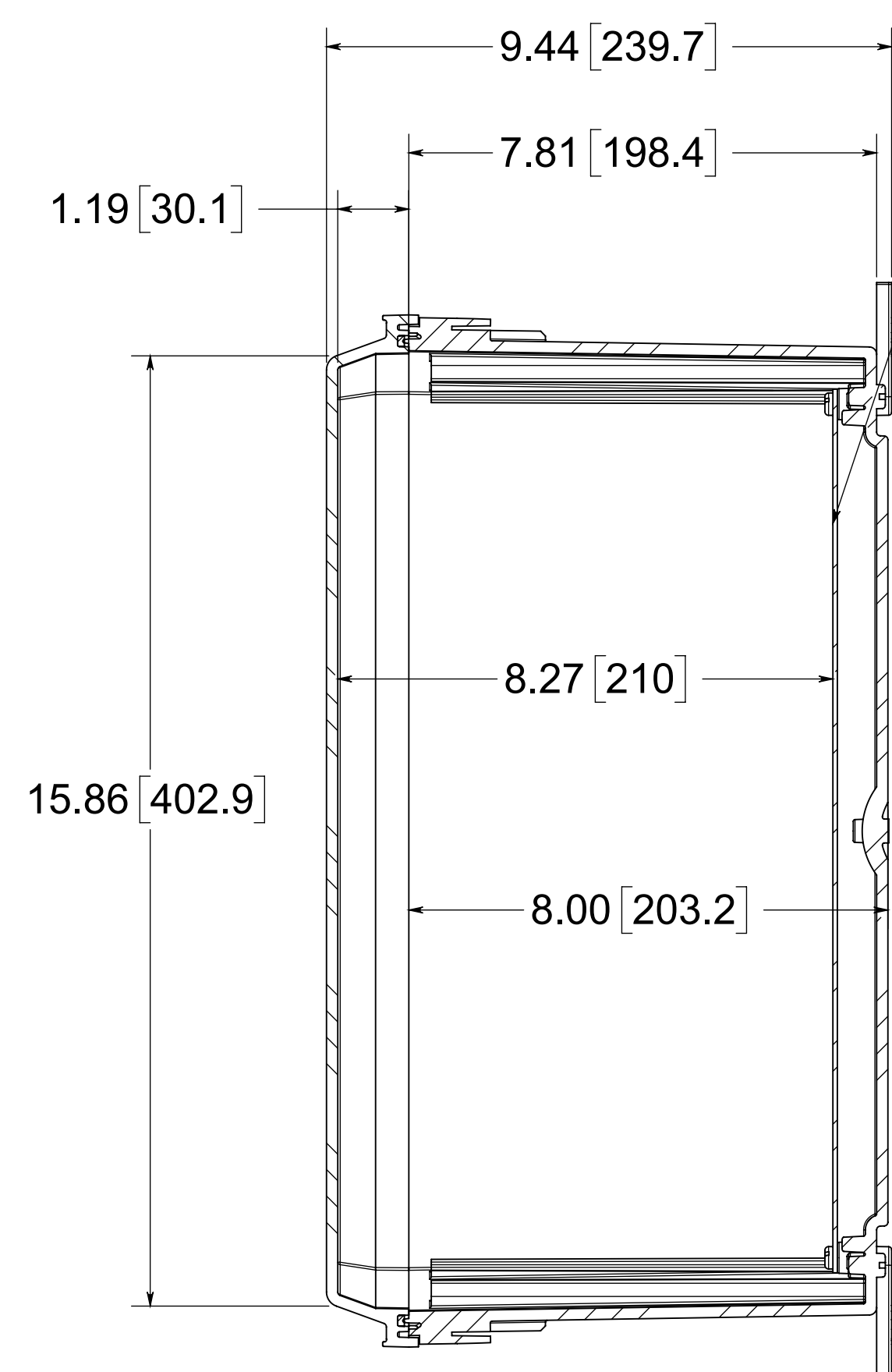
SECTION A-A
