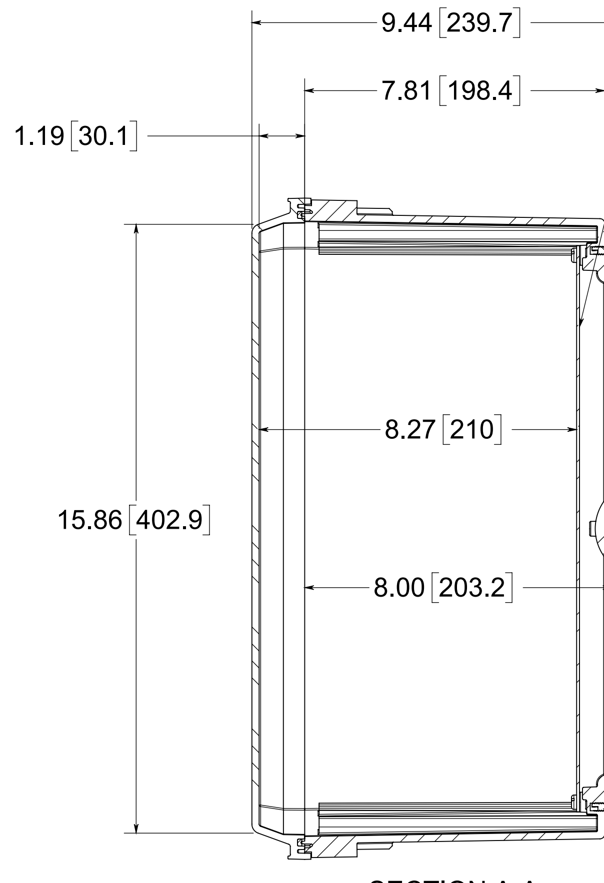
SECTION A-A
