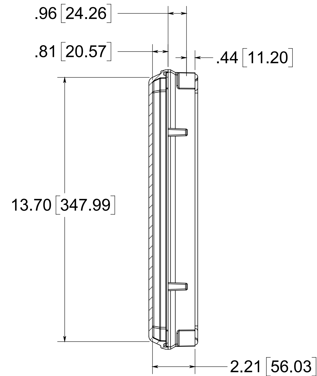
SECTION A-A
