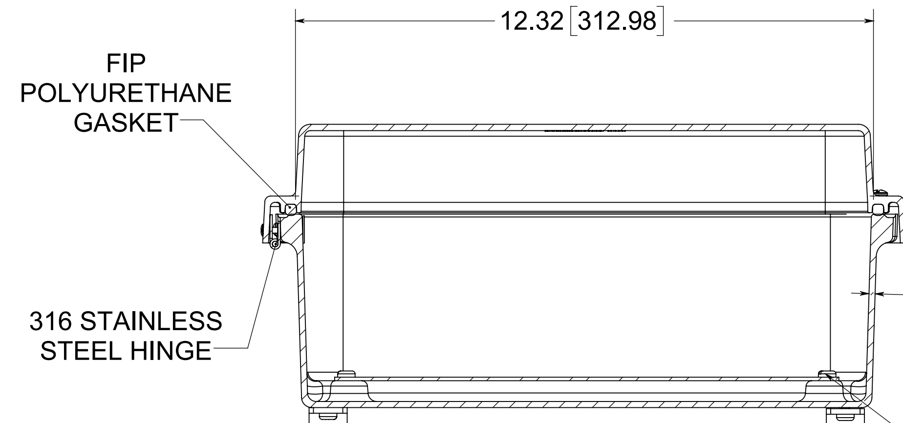
SECTION A-A
