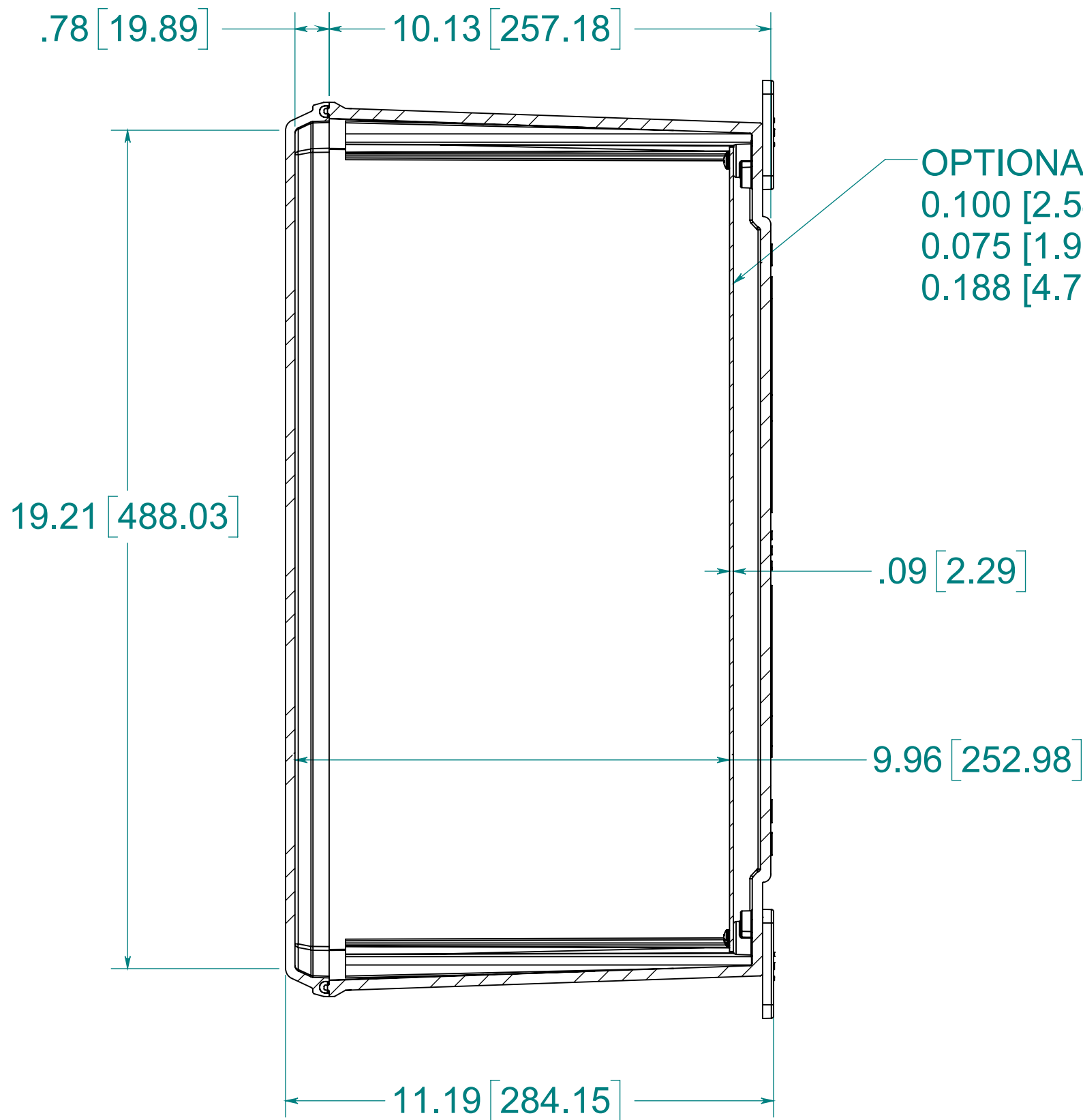
SECTION A-A
