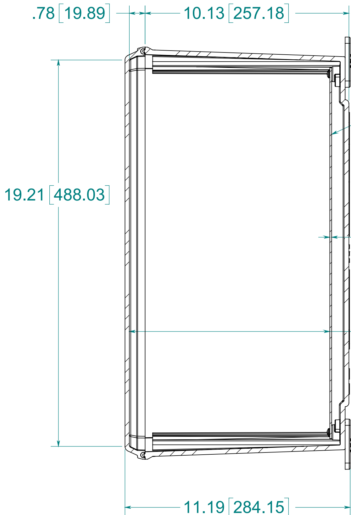
SECTION A-A
