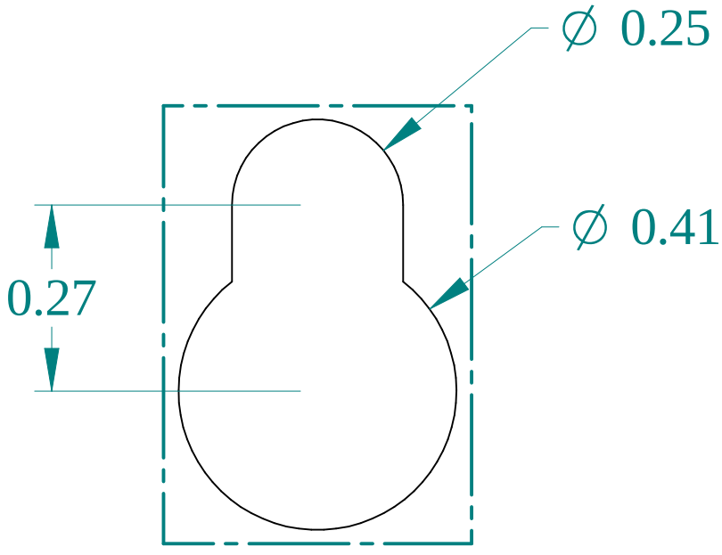
DETAIL Z TYP
