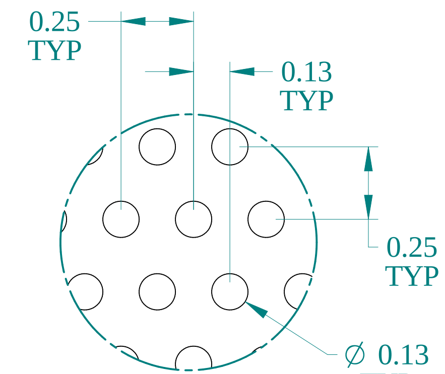
DETAIL Y
