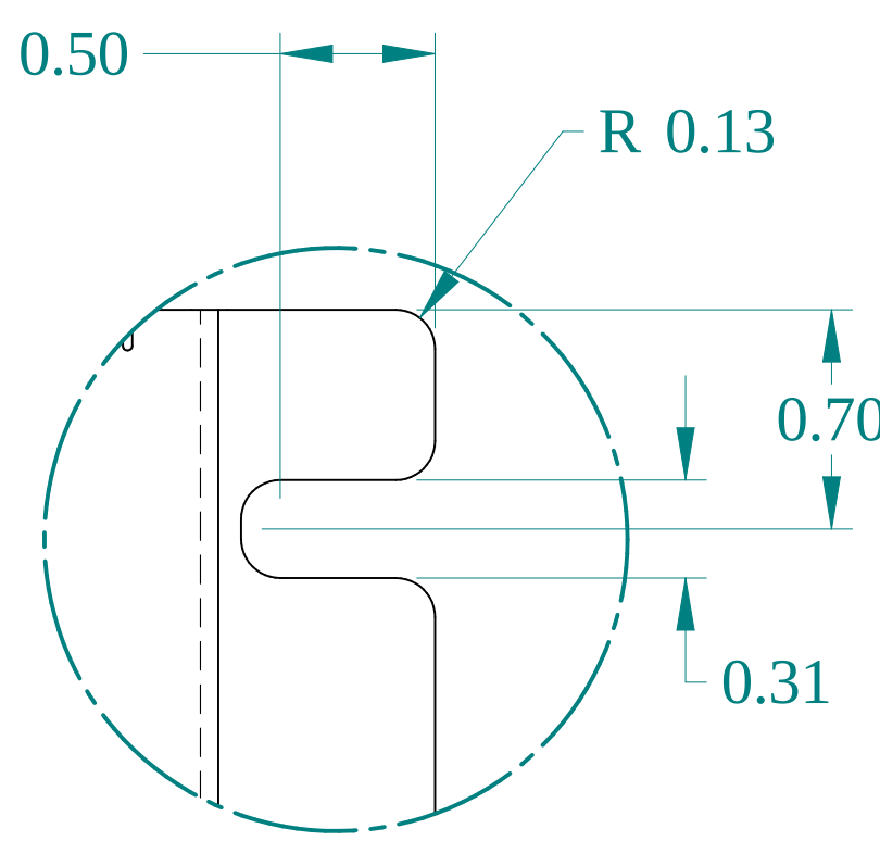
DETAIL Z TYP (4)
