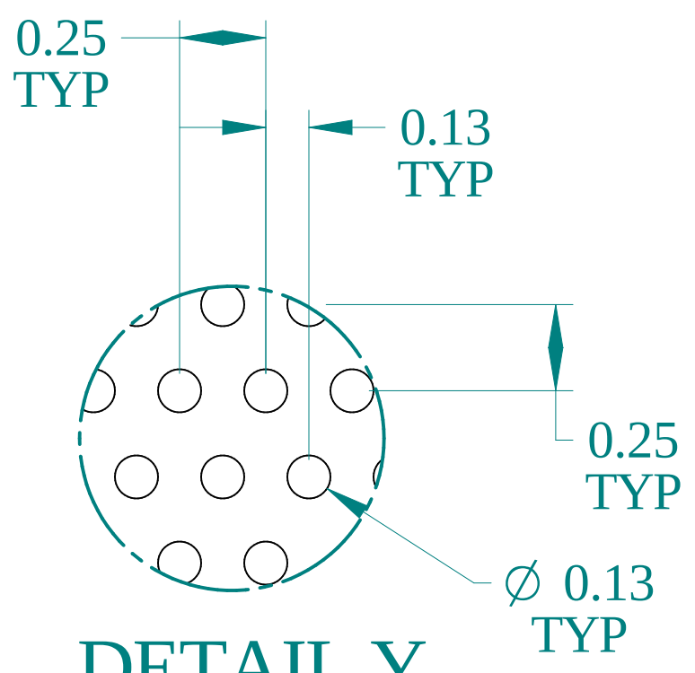
DETAIL Y
