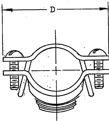
FIG. 1 MAT'L - STEEL
