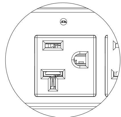
DETAIL A SCALE 1:1 TYP 8X
