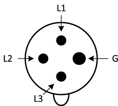
INPUT_PLUG_FRONT_VIEW
