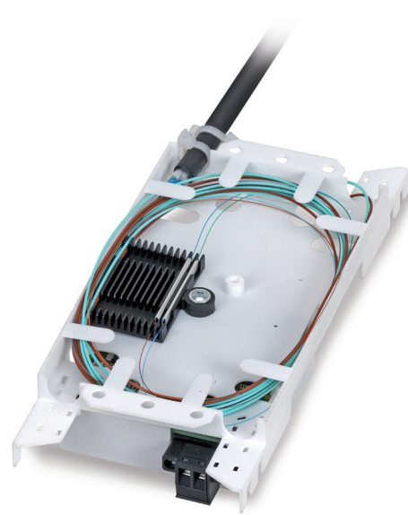
Spleißeinheit mit Spleißkamm und Pigtails
