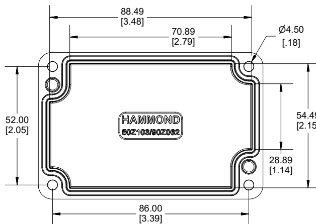
INSIDE LID
