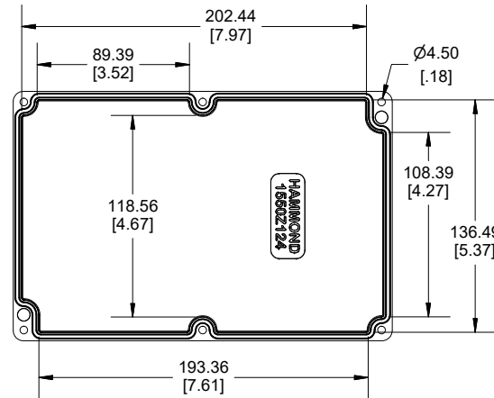
INSIDE LID
