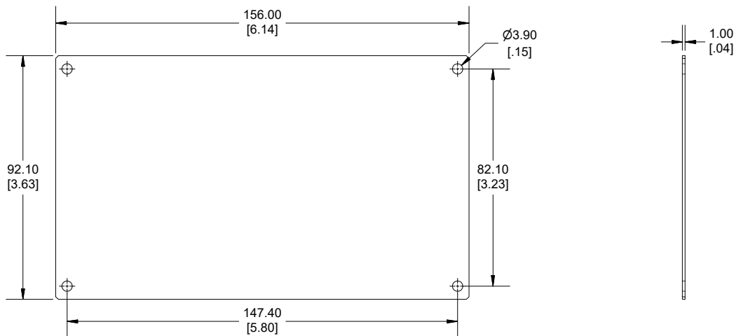
ENCLOSURE LID
