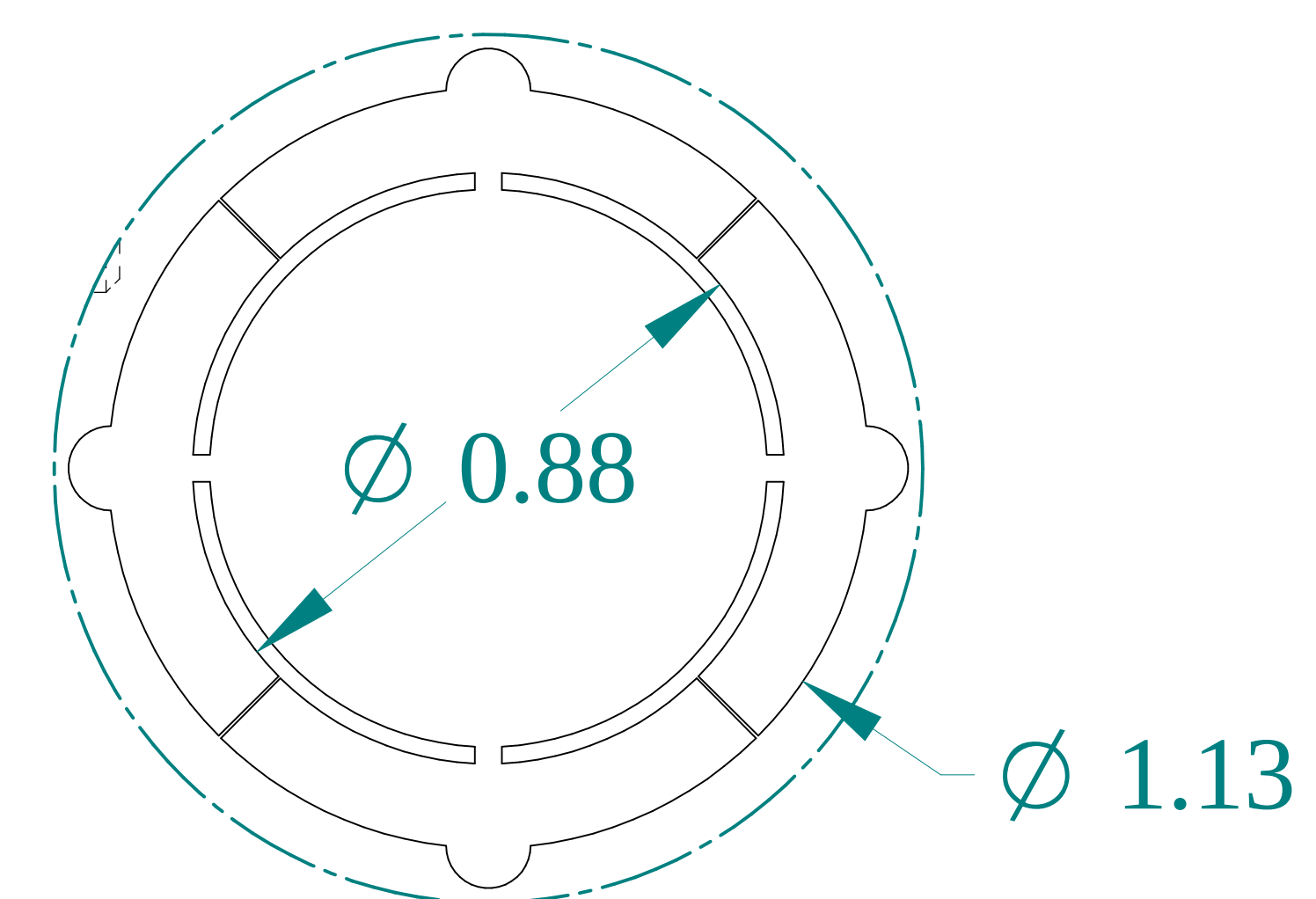
DETAIL Y
