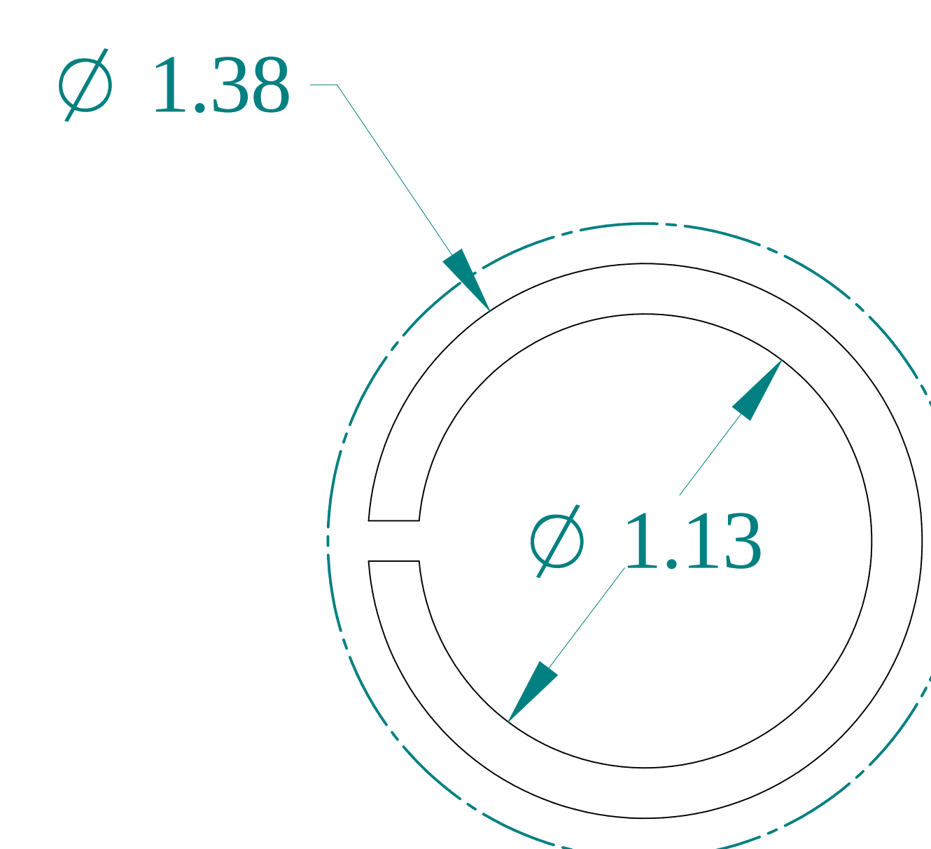
DETAIL Y
