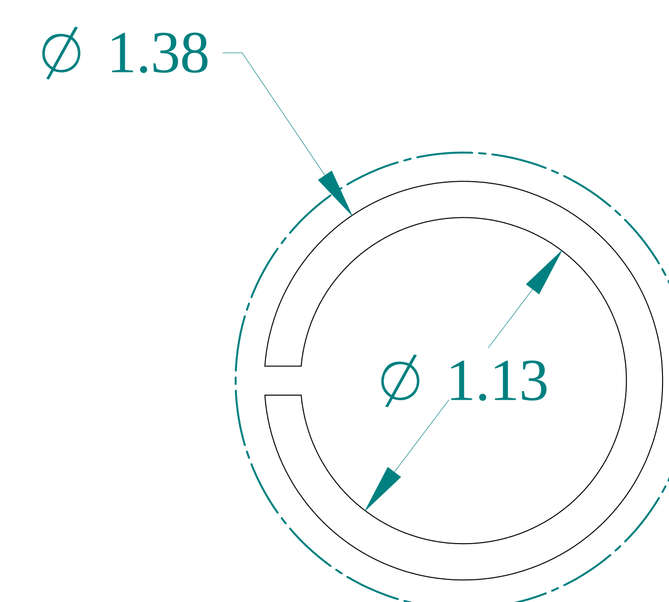
DETAIL Y
