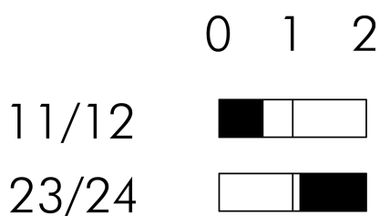
→ Schaltwegediagramm
