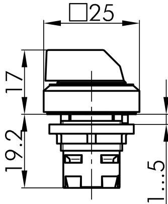
→ Maßskizze
