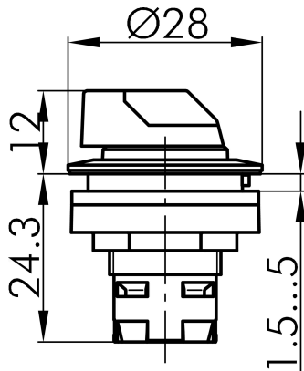
→ Maßskizze
