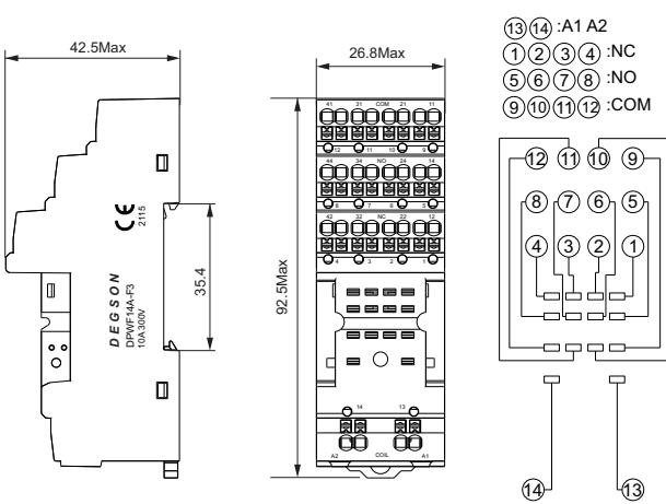
DPWF14A-F3
