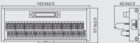
DM50-IDC-50-50-4Y-00Z(H)
