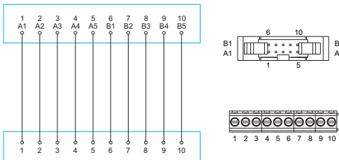
DM50-IDC-10-10-4Y-00Z(H)
