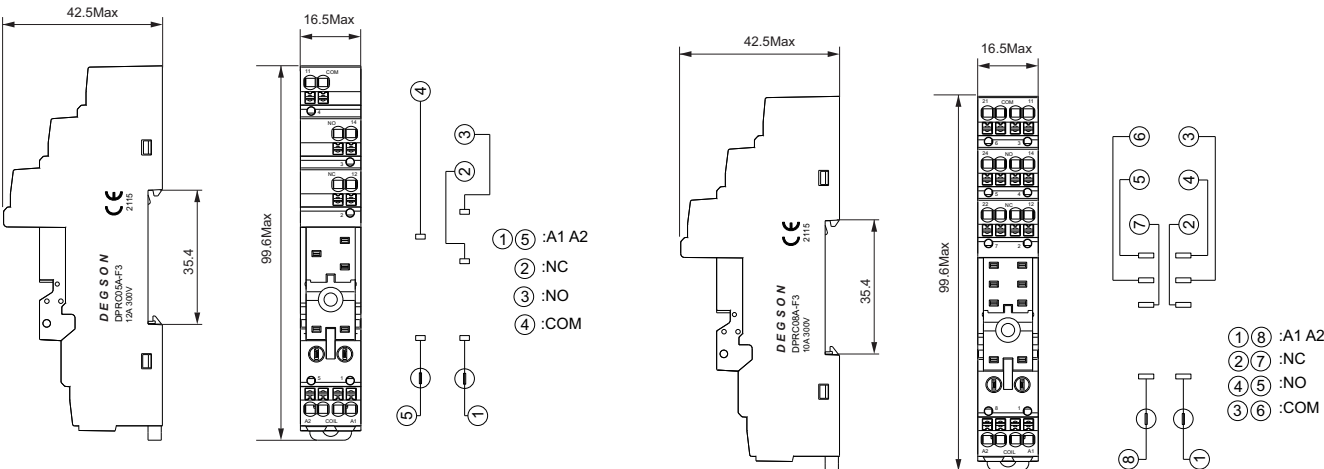
DPRC05A-F3
