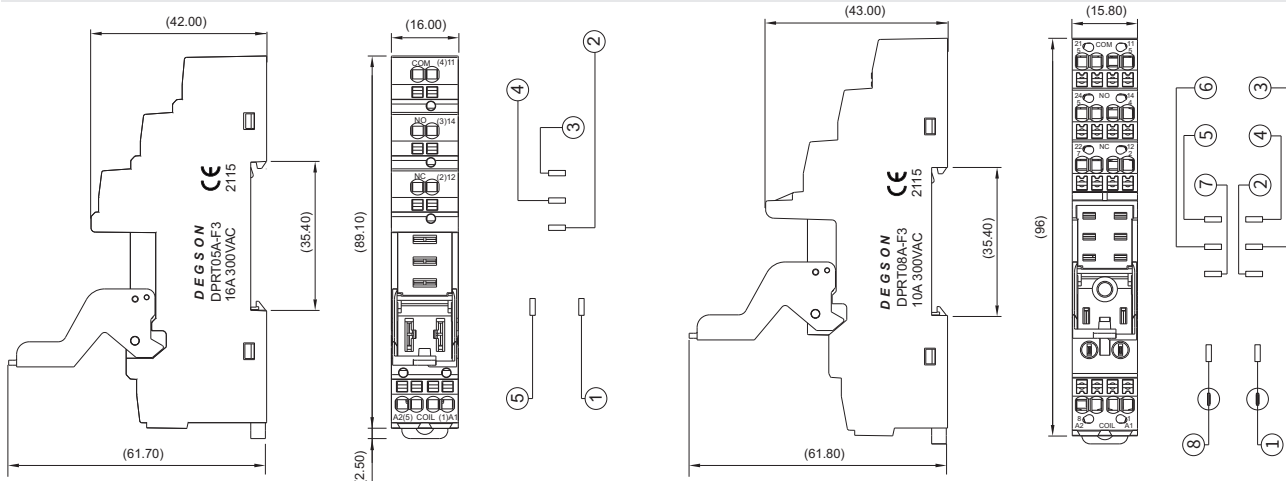
DPRT05A-F3
