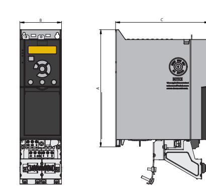
IP20/Open
